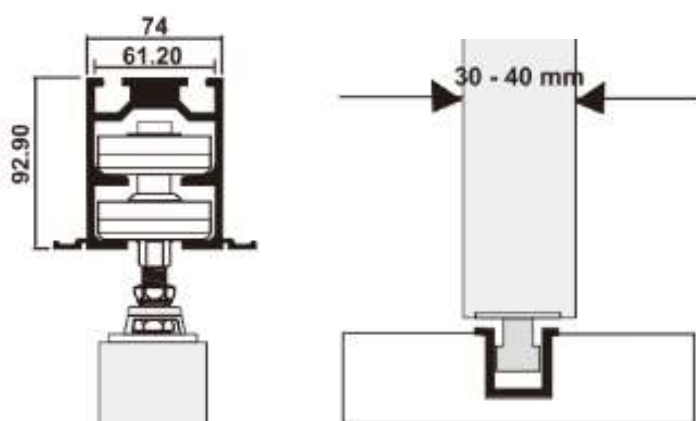
Edge Mount
