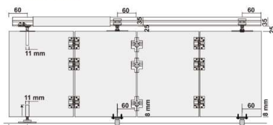
Edge Mount
