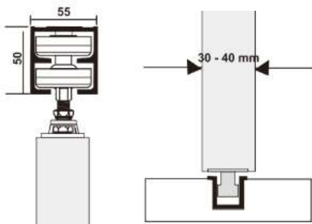
Edge Mount
